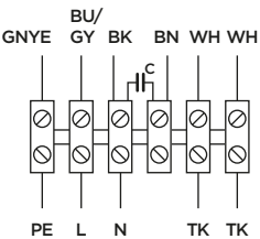
Схема № 3, 230 В, 1 ф
