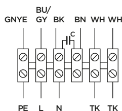
Схема № 3, 230 В, 1 ф
