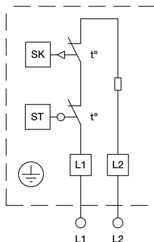
Схема 2 (400 В, 2 ф.)
