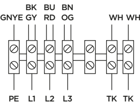
Схема № 5, 400 В, 3 ф
