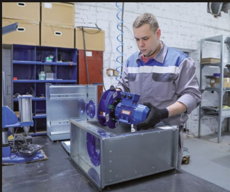
Производство элементов сборной вентиляции
