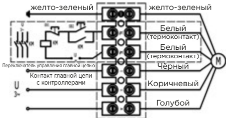
Схема № 2, 230 В, 1 ф
